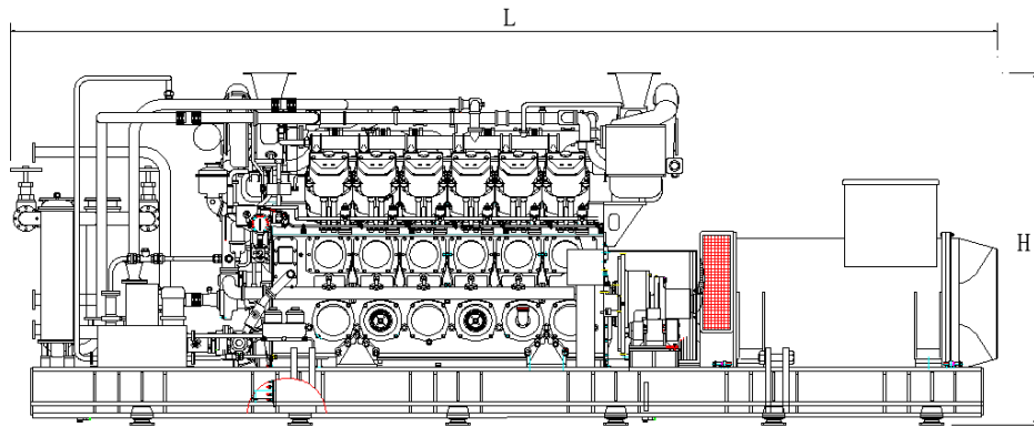
侧视图
