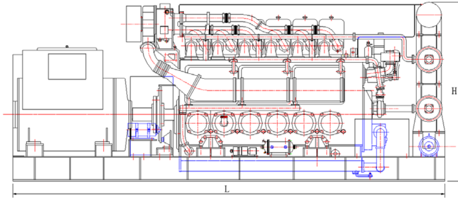
侧视图
