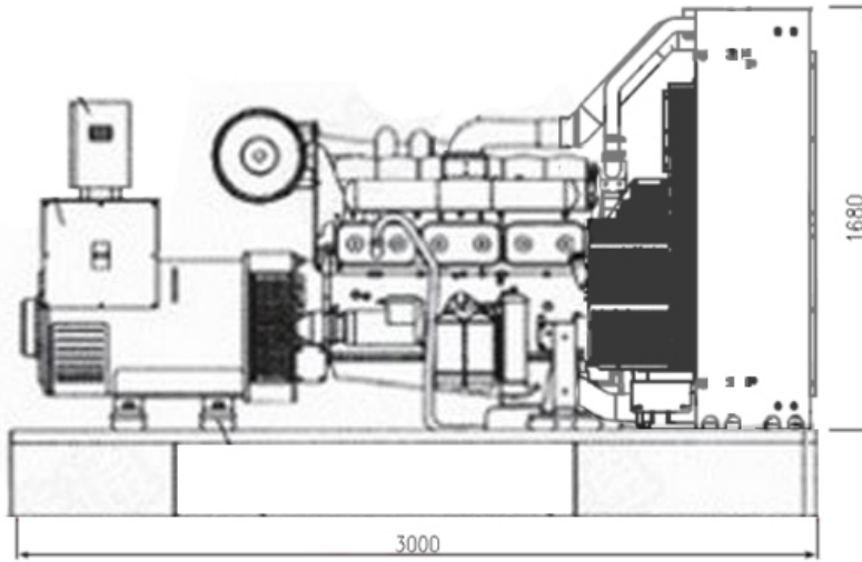
CPG300F8 机组侧视图
